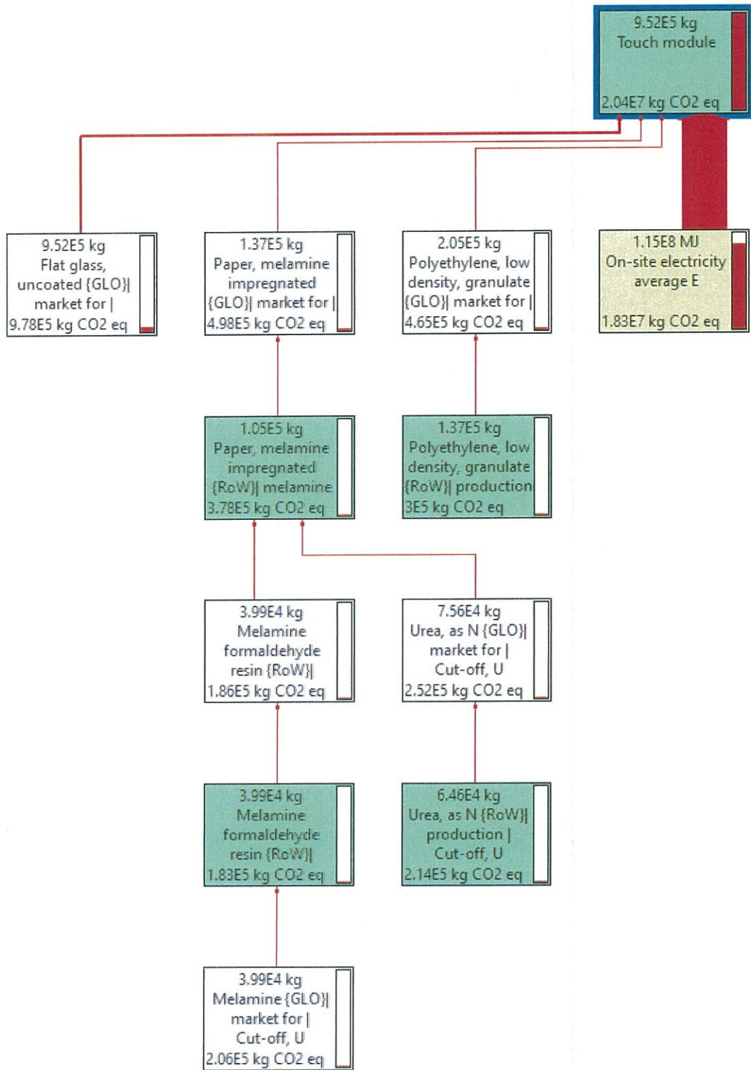
图5.2 touch module1生命周期建模总图
