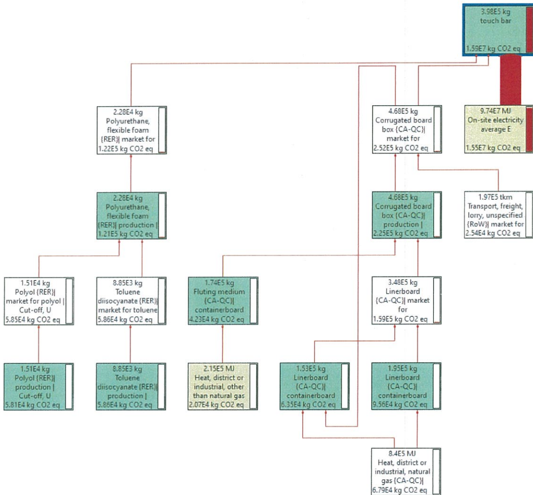
图5.1 touch bar生命周期建模总图
