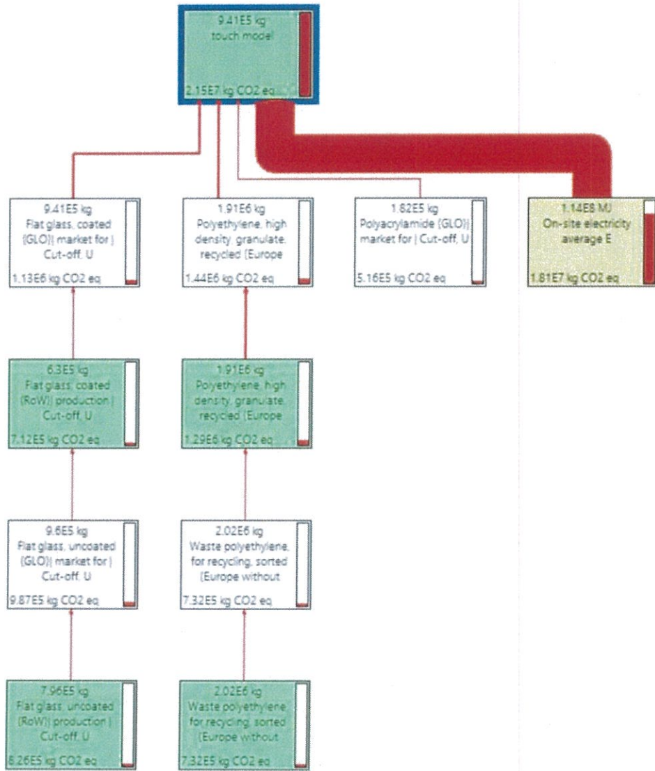
图5.3 touch module2生命周期建模总图
